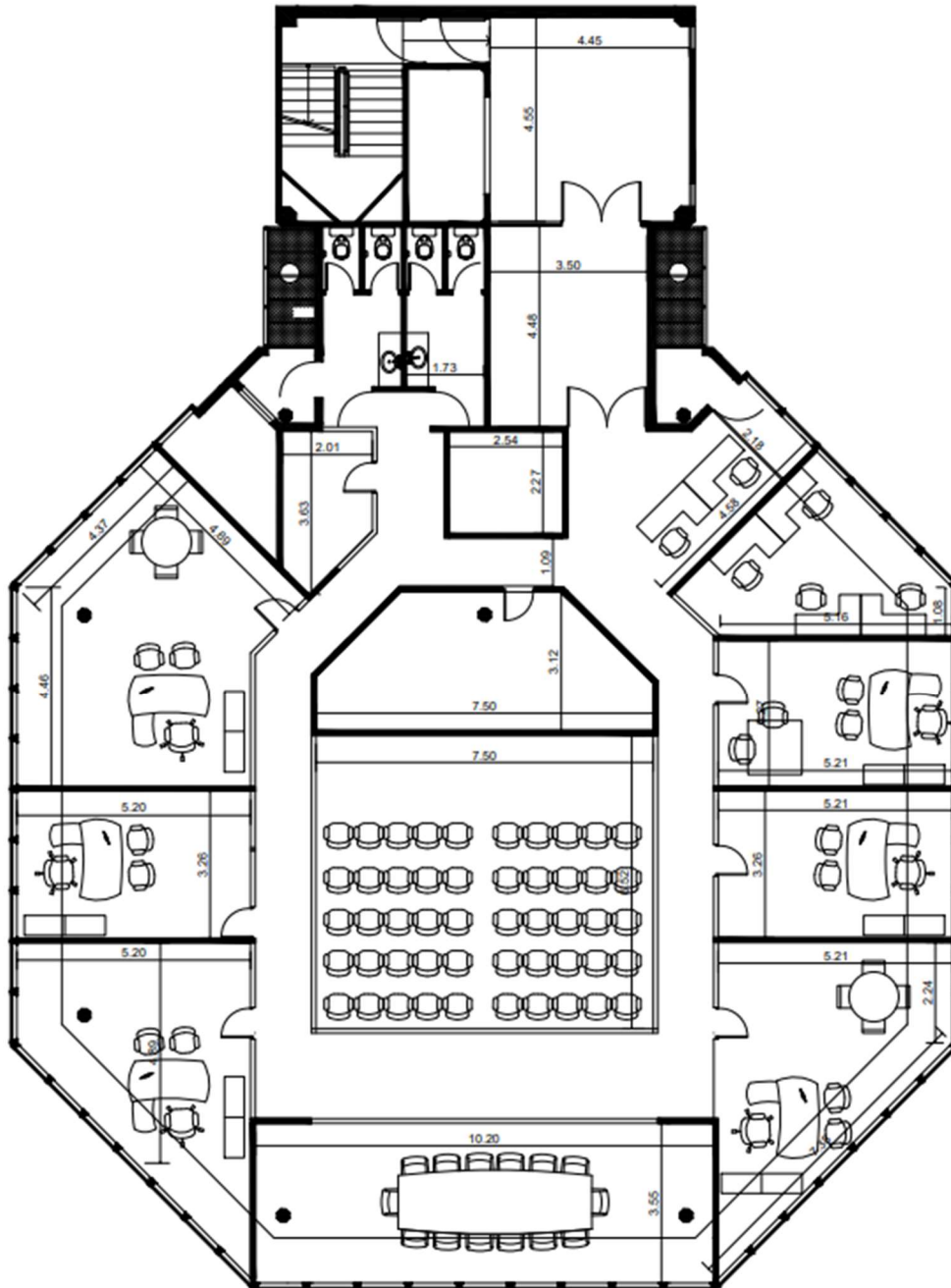
PLANTA 9º PISO
